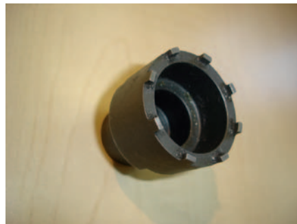
Tretlagerabzieher (2 vers.)
